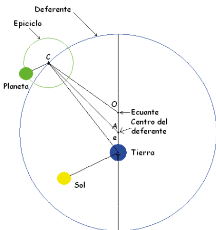
Figura 2. El modelo cosmológico instrumentalista de Ptolomeo en el Almagesto . En el Almagesto de Ptolomeo, el punto ecuante es el punto O, simétrico del punto T donde se halla la Tierra. La velocidad angular con que gira el planeta en el epiciclo es igual a la del Sol alrededor de la Tierra.
